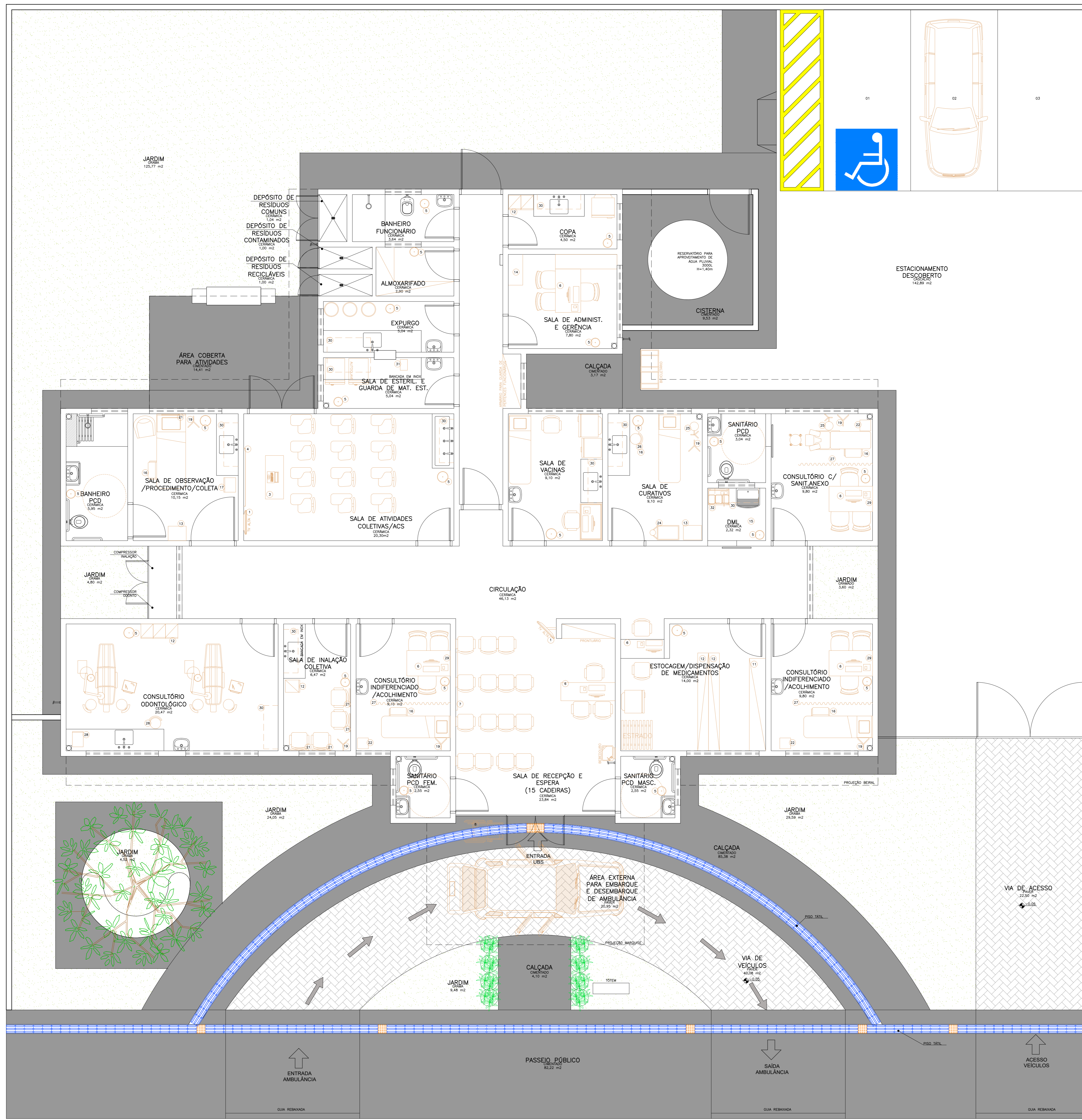
Planta Baixa Layout Nível: 0,00m Esc.: 1:50 Área: 288,22m 2
