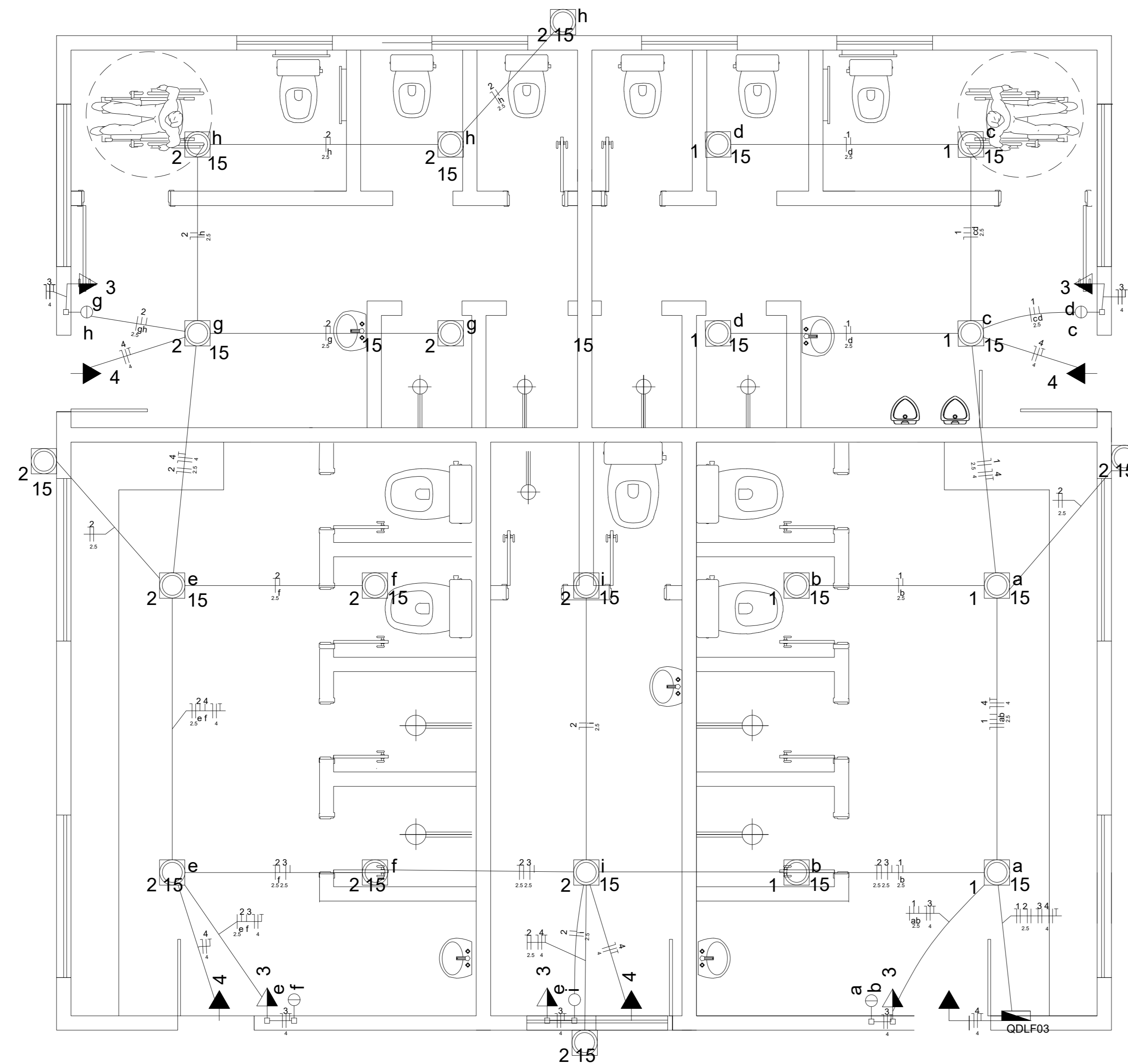
INSTALAÇÃO ELÉTRICA ILUMINAÇÃO E TOMADA VESTIÁRIO PAV. TERREO ESC. 150
