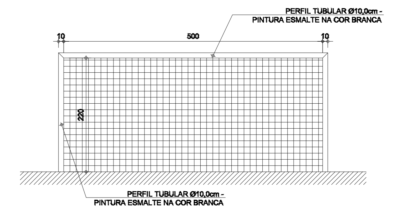
ELEVAÇÃO DAS TRAVES DO GOL ESCALA.....1/50
