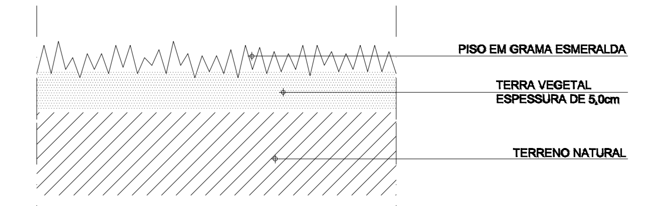
CORTE ESQUEMÁTICO PISO EM GRAMA ESCALA.....1/5
